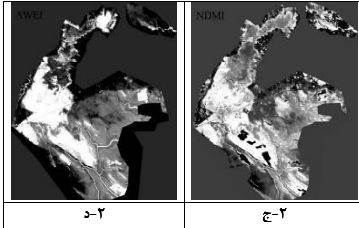
شکل ۲: حدود تالاب شناسایی شده از طریق شاخص‌های نرمال‌سازی آب لندست ۸ سال ۲۰۱۸.
